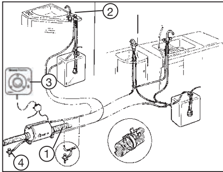
Schéma de l'alimentation en eau chaude
